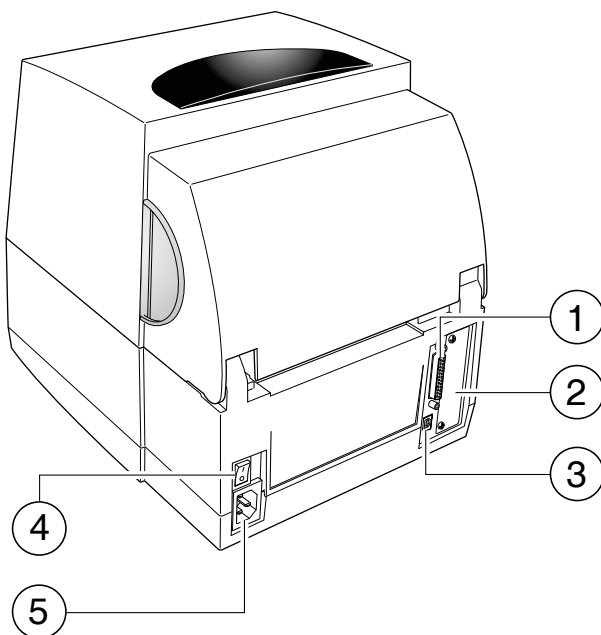
后视图
